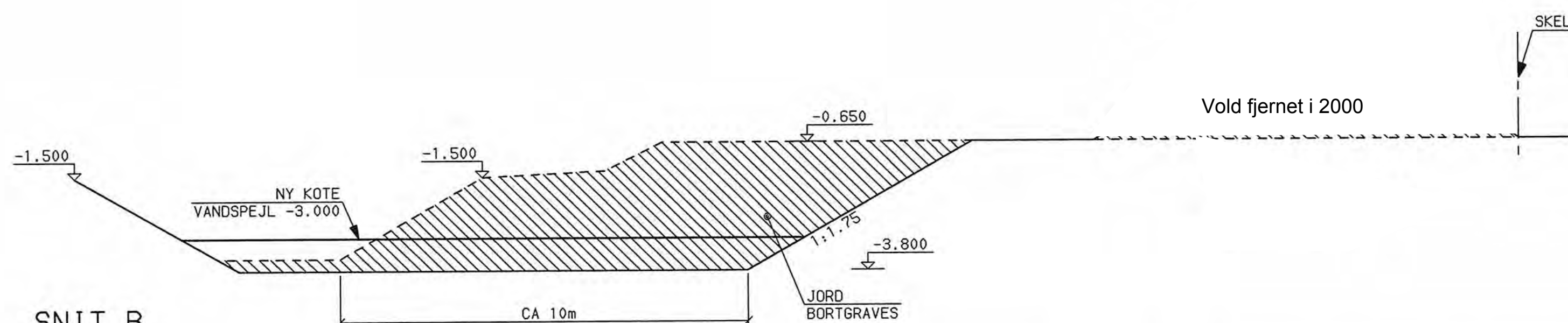
SNIT B 1:100
